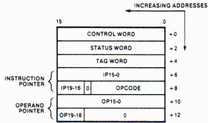
Figure 6-9. FSTENV and FLDENV Memory Layouts
